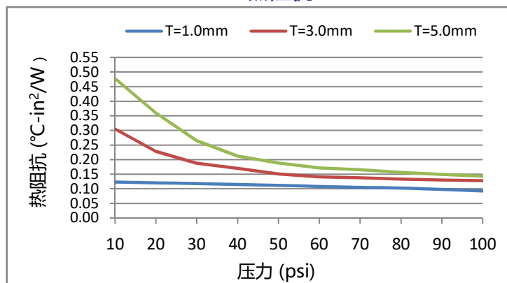
热阻抗
